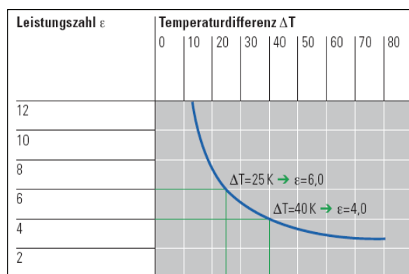
Abbildung 9: Leistungszahl \epsilon als Funktion der Temperaturdifferenz \Delta T zwischen Verdampfer und Verflüssiger ( T_0 = 273 \text{ K} ).
