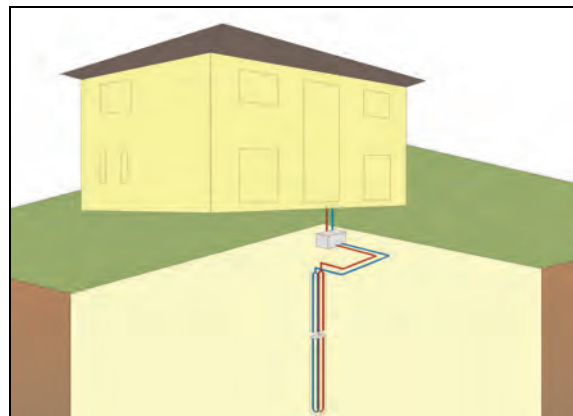
Abbildung 3: Schema Erdwärmesonde.
