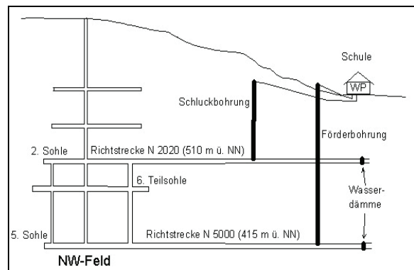
Abbildung 8: Schema Grubenwassernutzung der Zinngrube Ehrenfriedersdorf für die örtliche Mittelschule.
