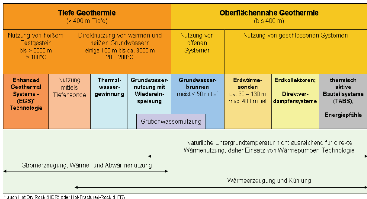
Abbildung 2: Übersicht Beispiele der Erdwärmenutzung.
