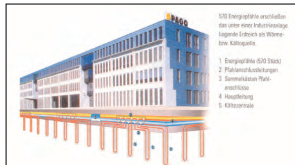
Abbildung 6: Schema erdberührte Betonbauteile.
